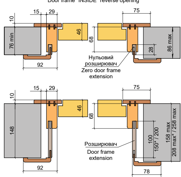
Короб "INSIDE" зворотного відкриття Door frame "INSIDE" reverse opening
