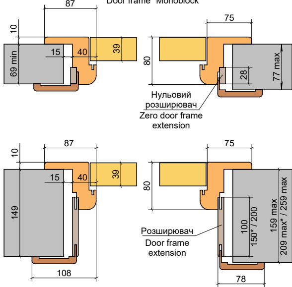
Короб "Моноблок" Door frame "Monoblock"
